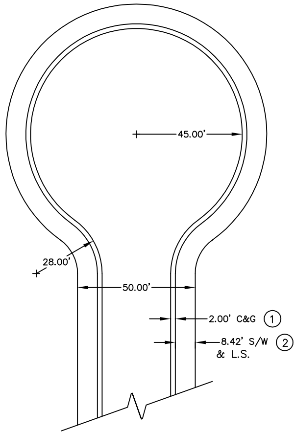
CUL-DE-SAC
